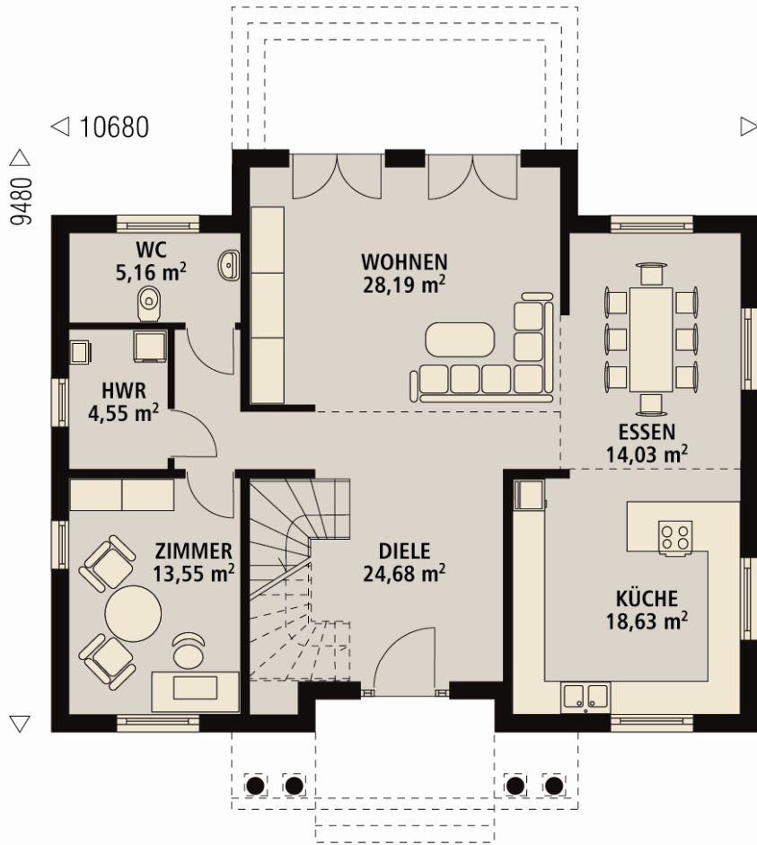
Erdgeschoss: 108,79 m 2
