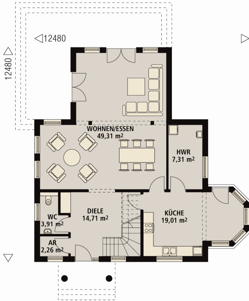
Erdgeschoss: 96,51 m 2
