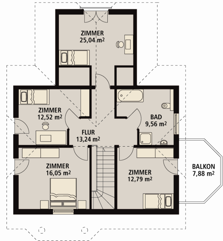
Dachgeschoss: 87,76 m 2
