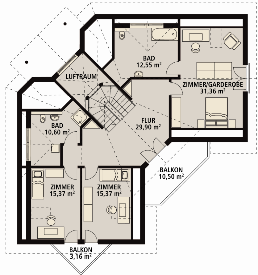
Dachgeschoss: 128,82 m²
